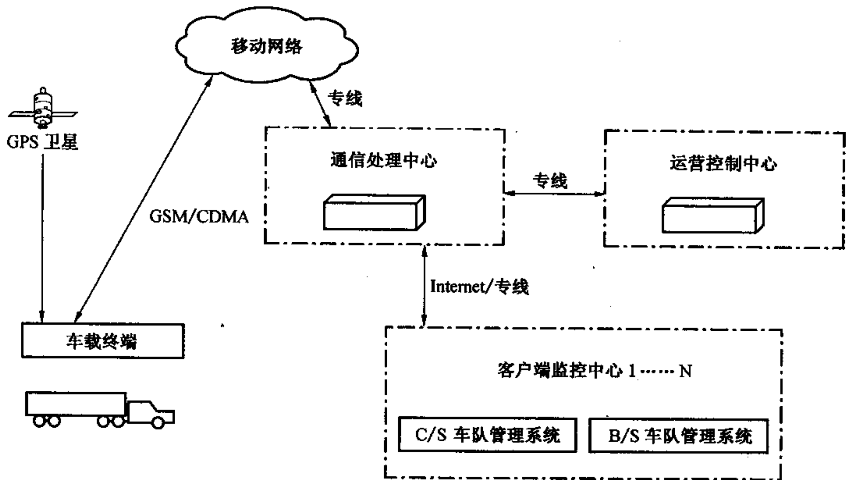
图 1 系统结构
